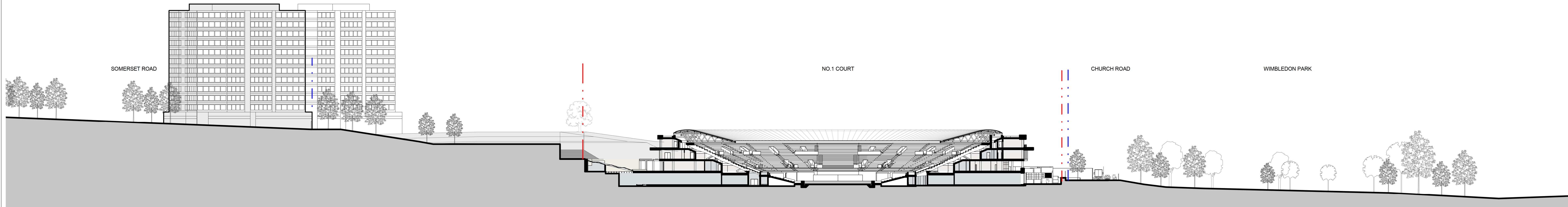
3 Site Section BB - Existing 1:500 0 5 10 25 50 m
